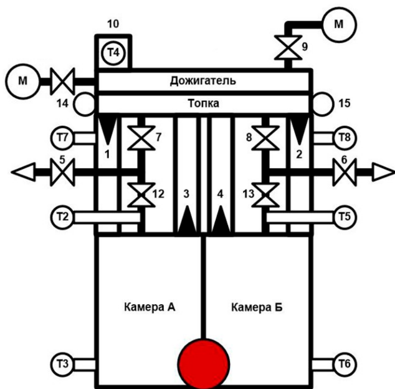
Схема органов контроля и управления печи
